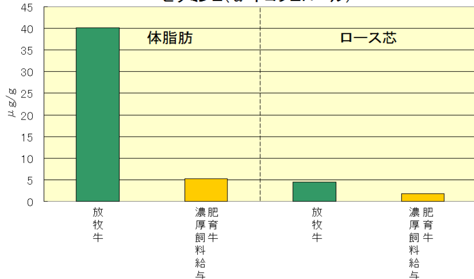
ビタミンE ( \alpha -トコフェロール)
