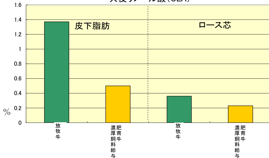
共役リノール酸 (CLA)
