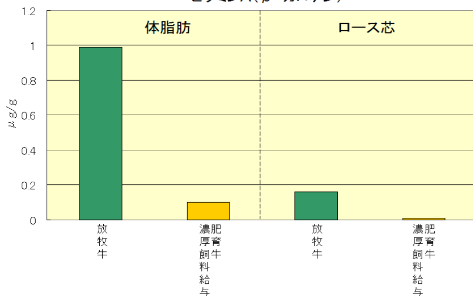
ビタミンA ( \beta -カロテン)
